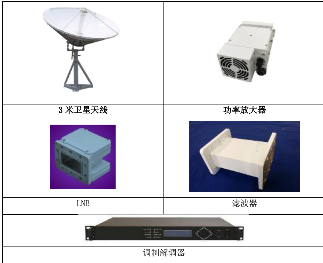
图 2-1 项目主要设备外观图
