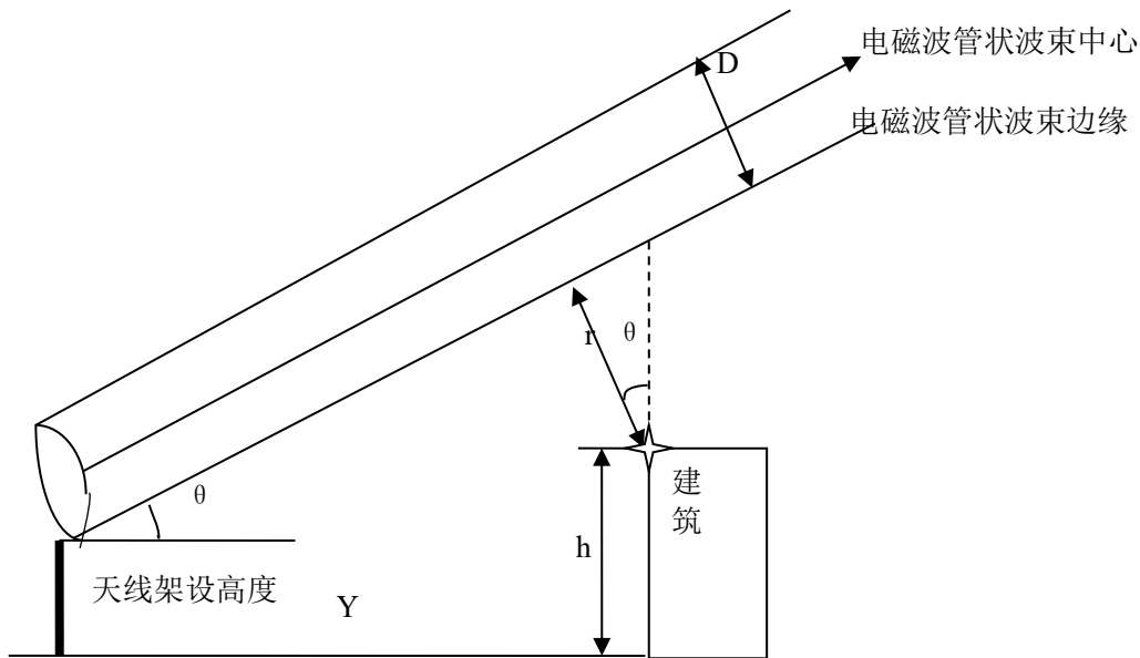
图 4-1 电磁辐射计算点离开管状波束的距离 r 示意图
