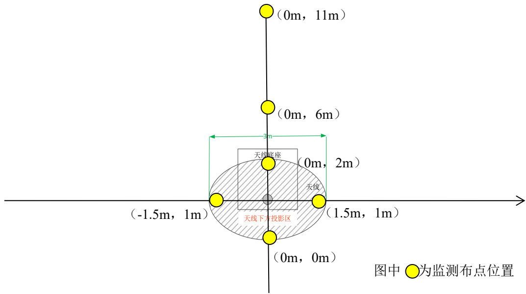
图 4-7 C 波段天线下方、背部类比监测示意图
