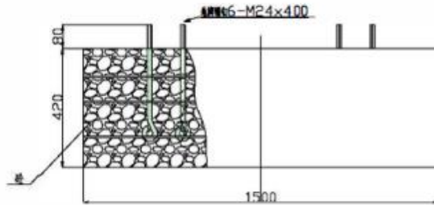
图 2-5 卫星天线基础结构示意图
