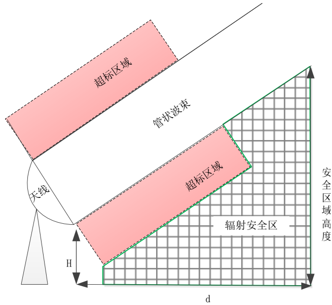
图 4-9 辐射达标防护区示意图
