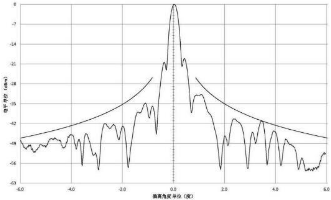
图 3-4 卫星天线方向性图
