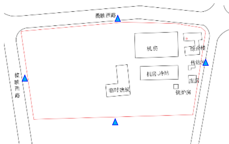
图 3-2 庙滩云联数据园区厂界处声环境监测布置图
