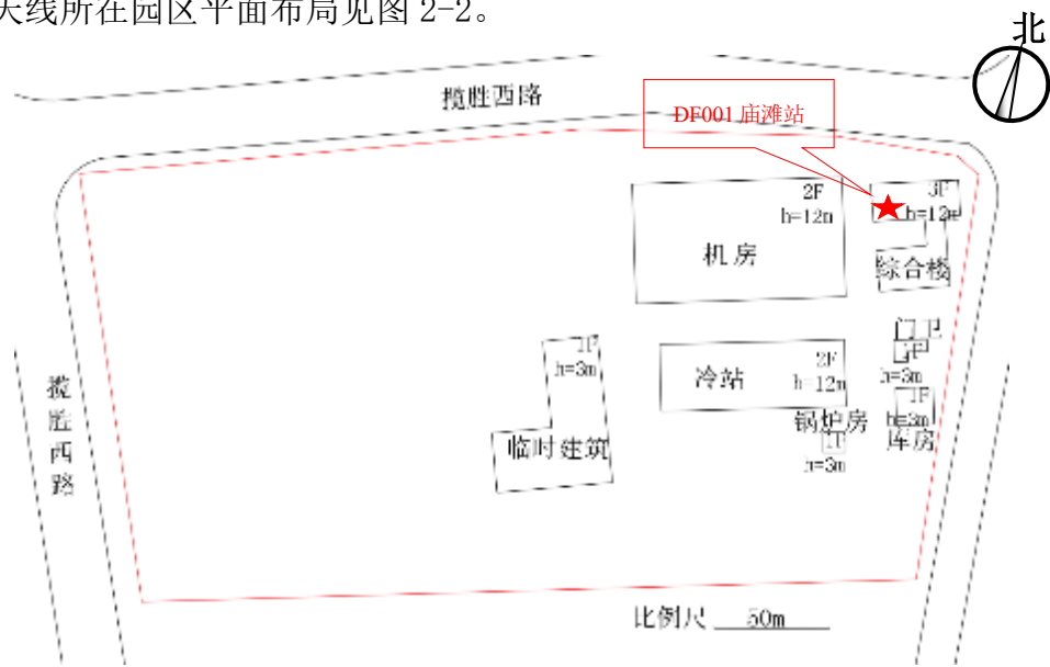
图 2-2 云联数据园区平面布局示意图
