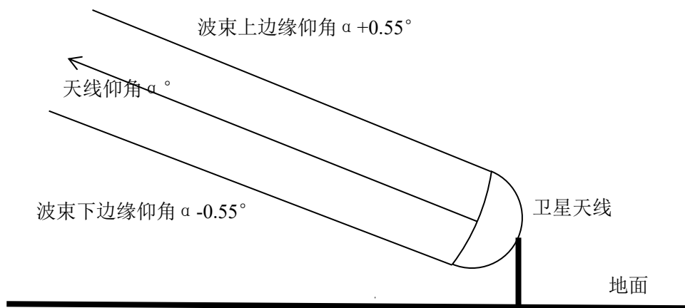
图 3-5 天线管状波束示意图（半功率角以 1.1° 计）
