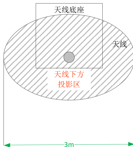
图 4-6 卫星天线下方、背面区域立面及平面示意图
