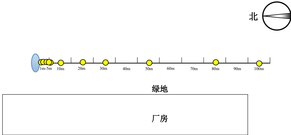
图 4-4 类比监测布点路径图
