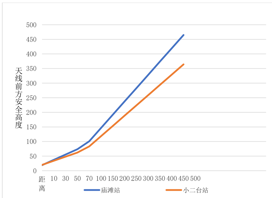
图 4-10 天线前方安全高度变化图
