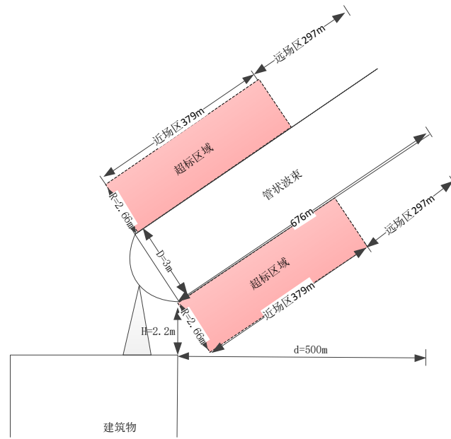
图 4-2 C 波段卫星天线额定功率运行时轴外辐射超标区示意图
