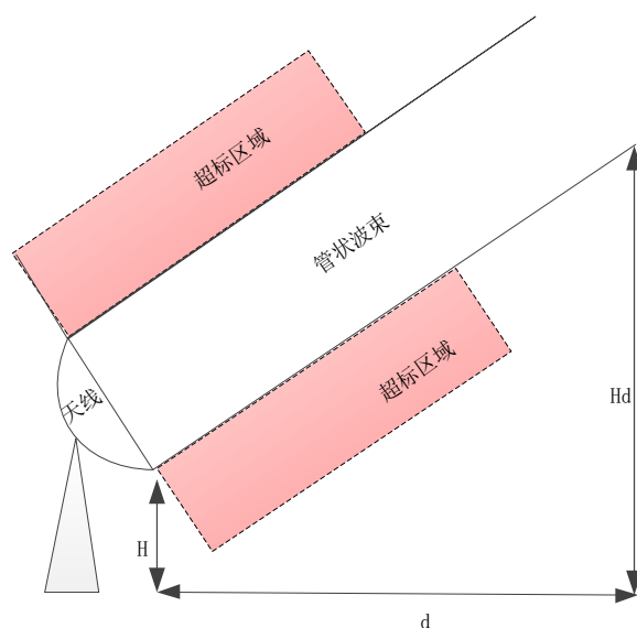
图 4-8 辐射达标区域示意图
